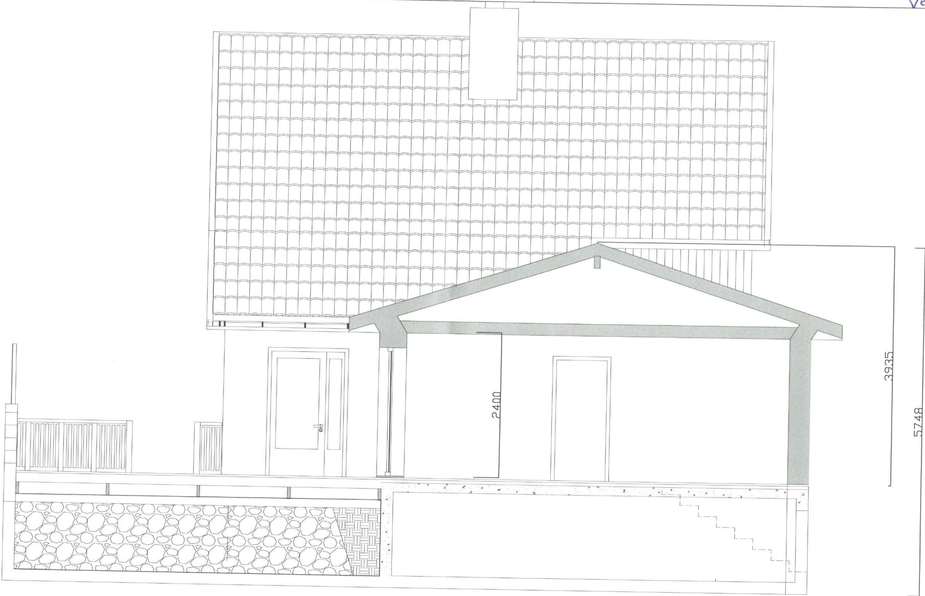
SNITT A-A
